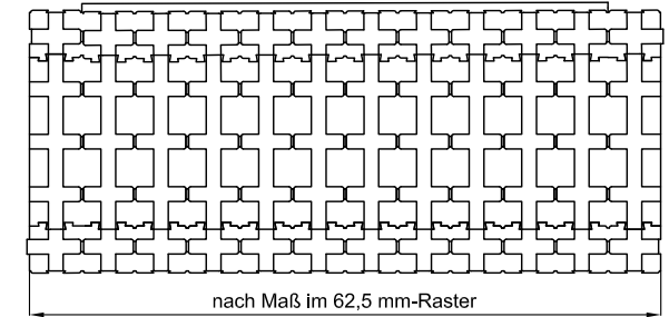
31er-Rollladenkasten, Revision außen, Rollraum 190 mm
