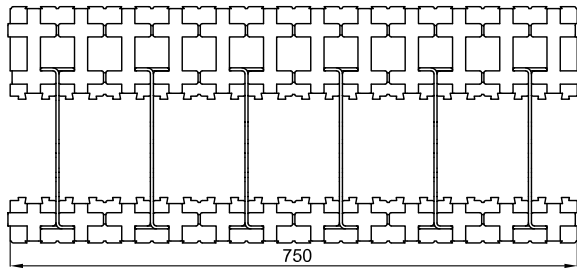
31er-Combielement
