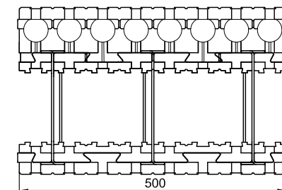
31er-Schalldämmelement
