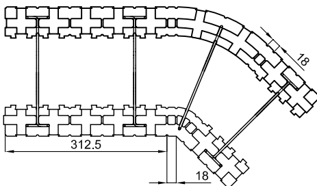
25er-Erkererlement 135° rechts (links o. Abbildung)
