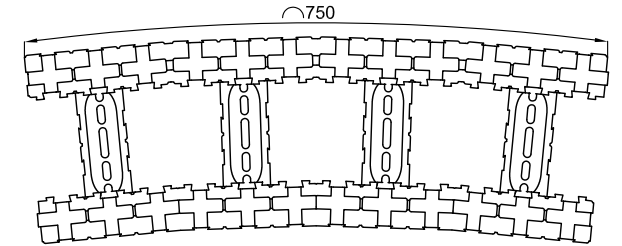
25er-Bogenelement, Radius nach Maß
