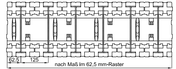
25er-Sturzelement 25 cm hoch
