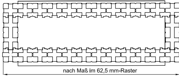
25er-Rollladenkasten, Revision innen, 160 mm Rollraum
