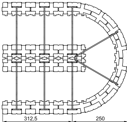
25er-Eckrundelement 180°
