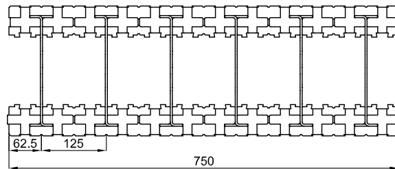
25er-Combielement
