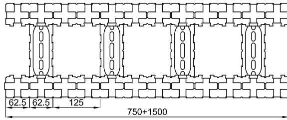
25er-Kompaktelement
