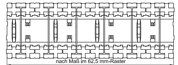
25er-Sturzelement 12,5 cm hoch
